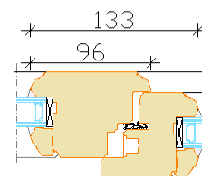
Mitteavatav osa, püstimpst ja avatav raam
