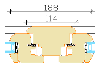
Avatavad raamid püstimpstiga
