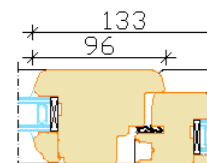
Avatav raam, püstimpost ja mitteavatav osa
