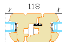
Pool-poollega avatavad raamid
