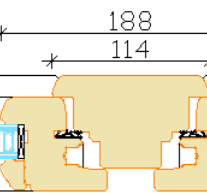
Avatavad raamid püstimpostiga
