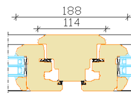
Avatavad raamid püstimpostiga
