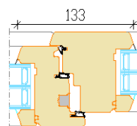
Avatav raam, püstimpost ja mitteavatav osa
