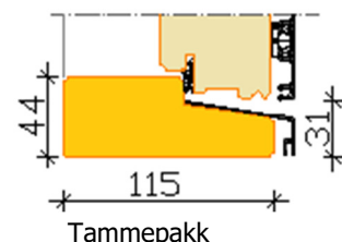
Combi lävepakk
