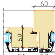
Püstimpost
