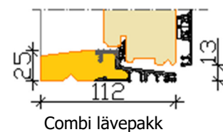
Alumiinium lävepakk
