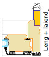
Leng + laiend
