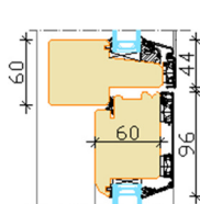
Rõhtimpost
