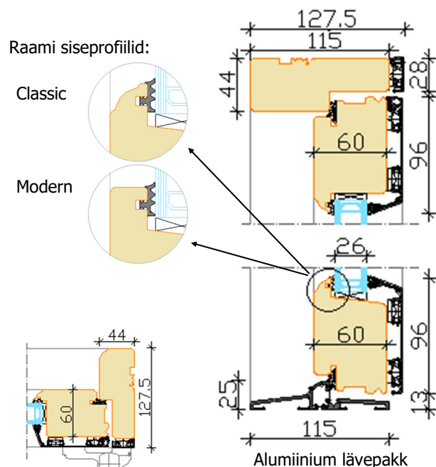
Standard leng
