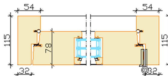
Standard jamb
