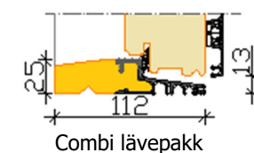
Alumiinium lävepakk
