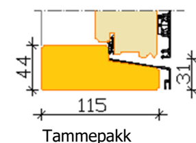
Combi lävepakk
