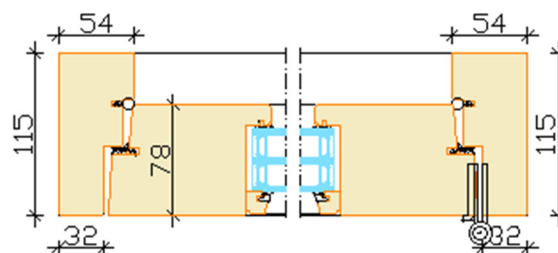
Standard jamb
